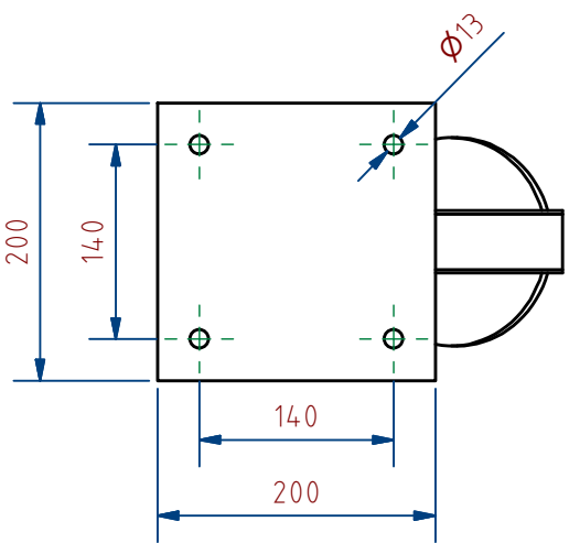
PLACA PARA ASIENTO ( 1 : 6 )
