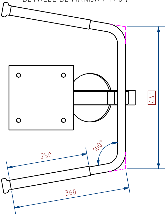
DETALLE DE MANIJA ( 1 : 6 )
